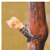
Otváranie pupeňov
